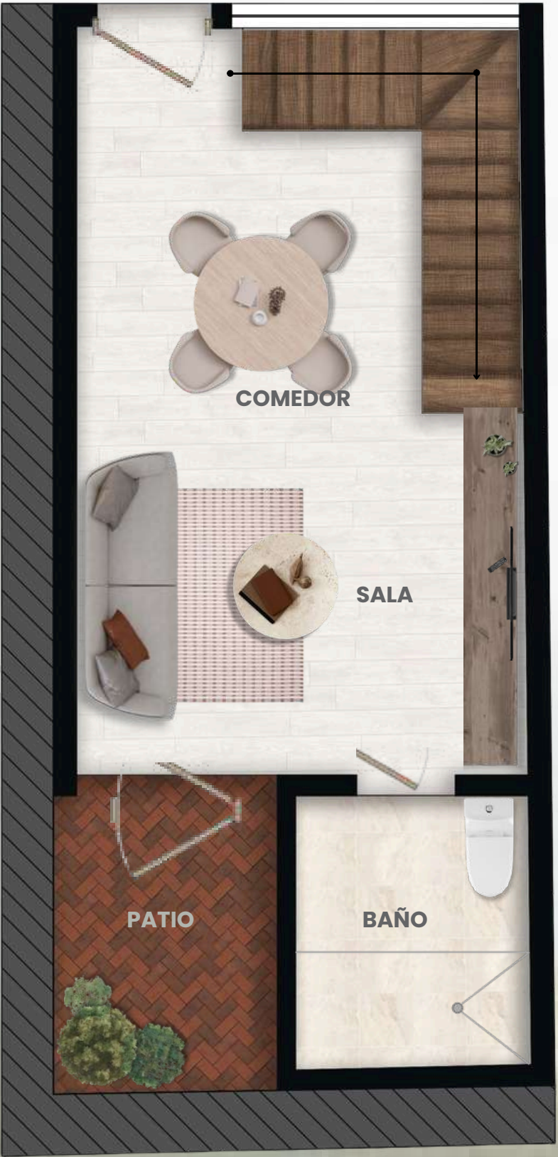
PLANTA BAJA
