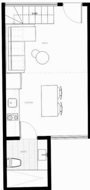
PLANTA BAJA
